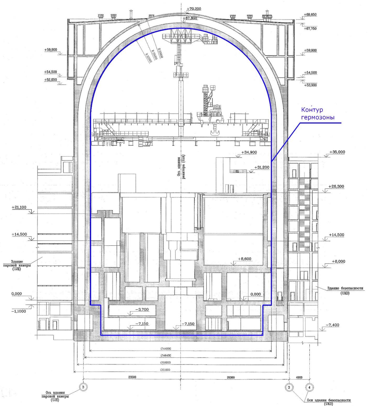
Рисунок 3. Здание реактора
