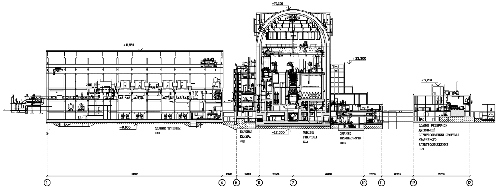
Рисунок 2 – Компонка основных зданий энергоблока. Разрез 1-1
