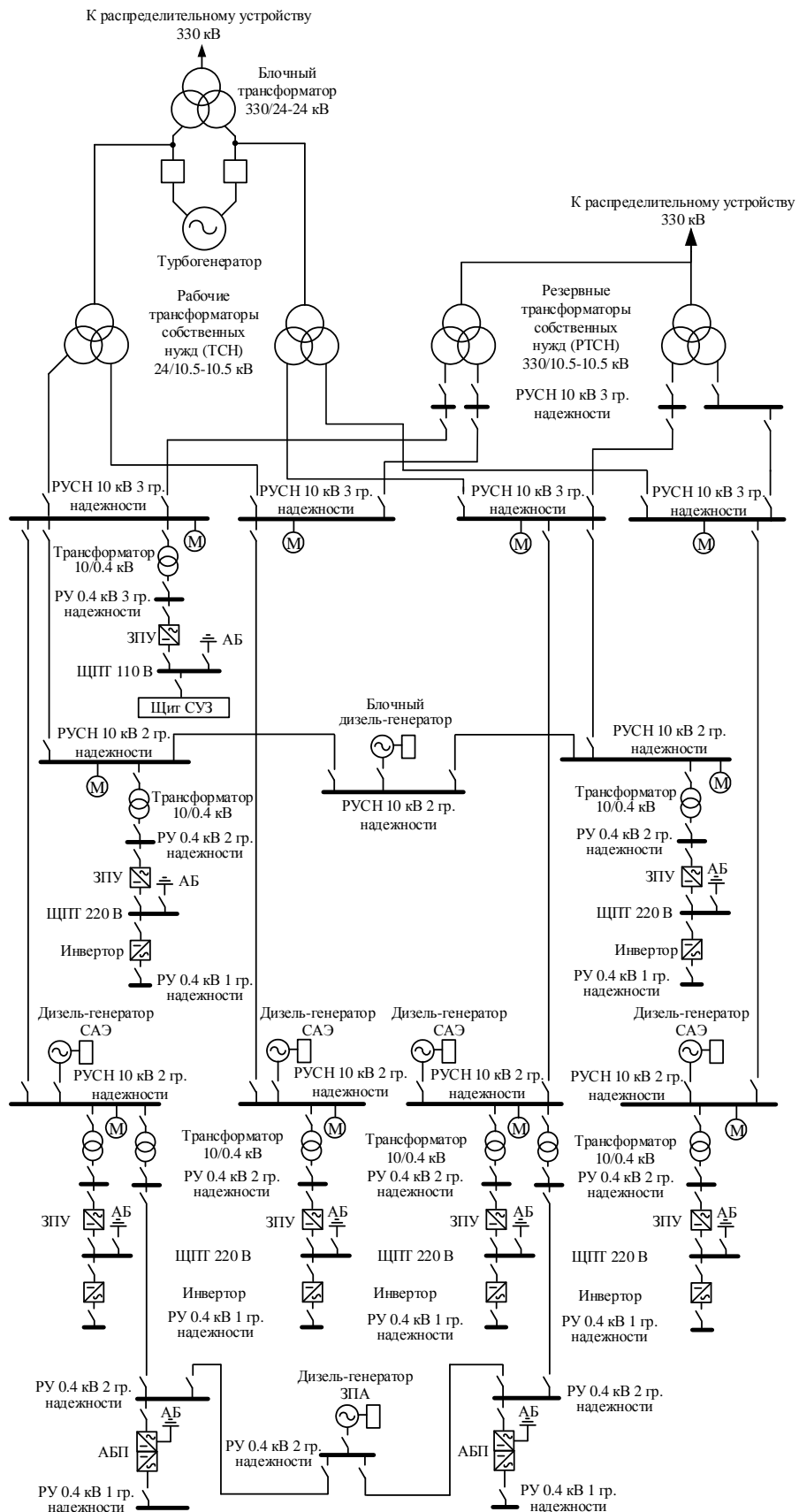
Рисунок 11.2.2.1 – Структурная схема электроснабжения собственных нужд АЭС
